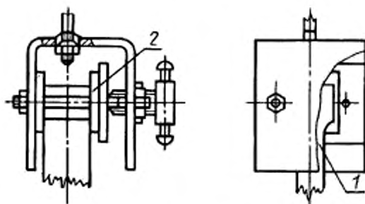
1 — образец; 2 — щечки захвата
