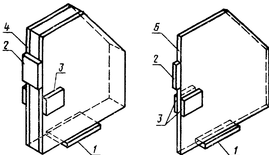
Схемы размещения подкладок и их установки
