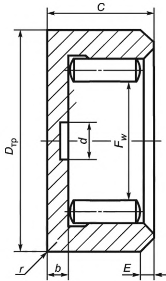
Рисунок 2 — Роликовый игольчатый карданный подшипник с фаской на наружном диаметре без галтели на донышке
