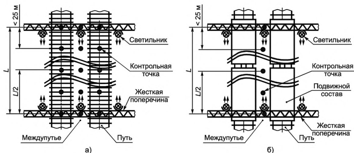
Рисунок 2 — Схема расположения контрольных точек измерения освещенности участка, освещаемого с жестких поперечин
