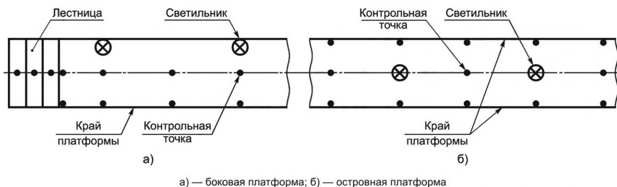
Рисунок 3 — Схема расположения контрольных точек измерения освещенности на платформах
