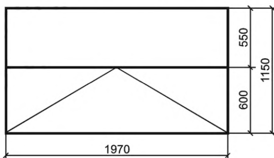
Рисунок 3 — Эскиз оконного блока
