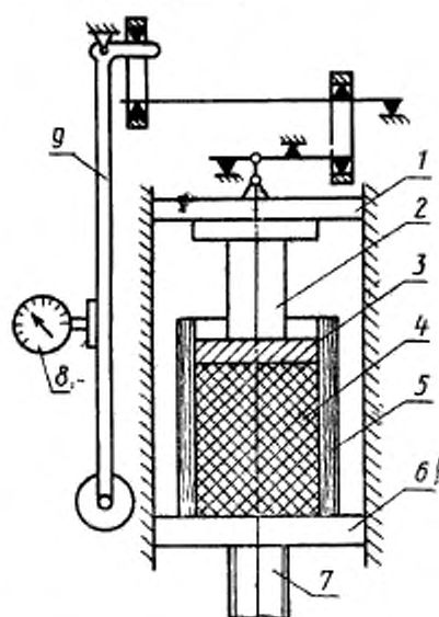
1—верхняя плита, 2—пуансон, 3—диск, 4—парафин, 5—втулка, 6—нижняя плита, 7—винт, 8—измеритель усилия, 9—мантия
