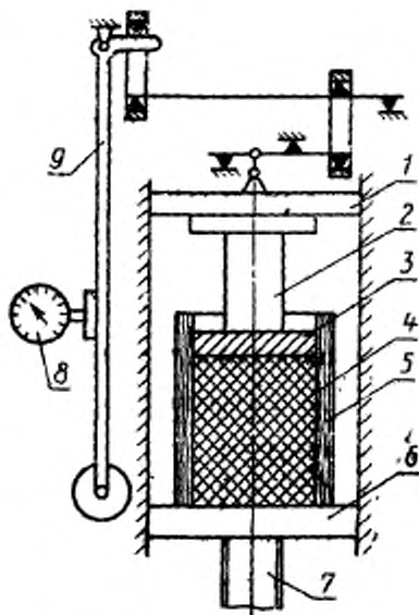
1 — верхняя плита; 2 — пуансон; 3 — диск; 4 — парафин; 5 — втулка; 6 — нижняя плита; 7 — шпиг; 8 — измеритель усилия; 9 — маятник
