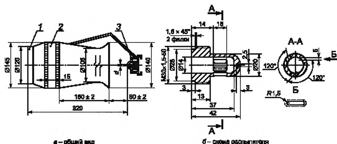
1 — корпус; 2 — пакет сеток; 3 — распылитель
