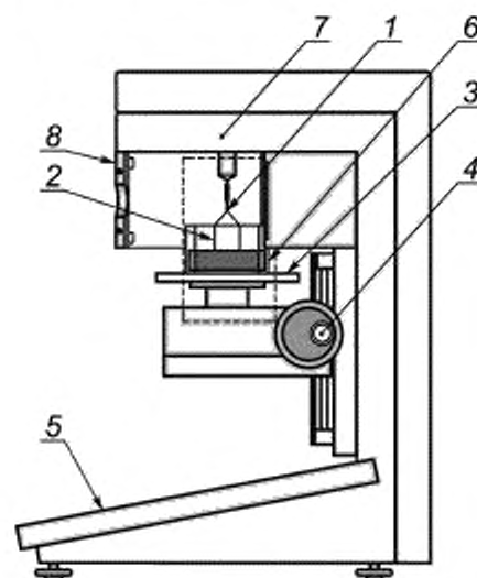
1 — измерительное кольцо; 2 — плечо измерительного кольца; 3 — горизонтальная платформа тензиометра; 4 — ручка подъемного механизма столика; 5 — панель управления тензиометра; 6 — кювета с рабочим раствором; 7 — весовая система; 8 — защитный экран
