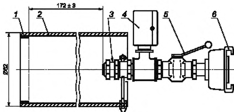
1 — сетка; 2 — корпус; 3 — распылитель; 4 — манометр; 5 — кран; 6 — соединительная головка
