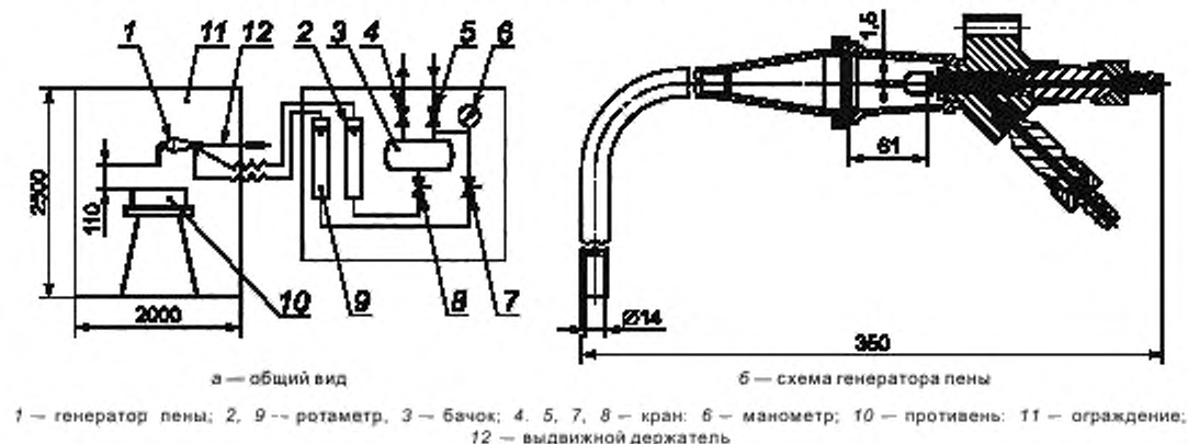
Рисунок 6 — Схема установки для тушения пеной средней кратности (стендовая методика)
