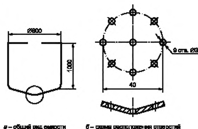
Рисунок 5 — Емкость для сбора пены
