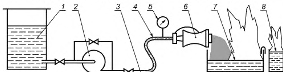
7 — емкость с рабочим раствором пенообразователя; 2 — насос; 3 — трубопровод; 4 — рукав; 5 — манометр; 6 — пожарный ствол; 7 — противень; 8 — тигль
