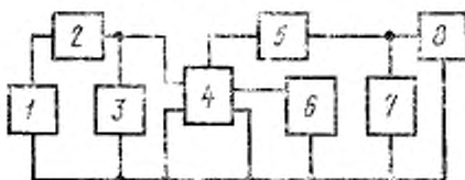
1—генератор постоянного напряжения (тока); 2, 5—измерители постоянного тока; 3, 8—изме- рители постоянного напряжения; 4—переключа- тель; 6—нагрузка; 7—блок питания.
