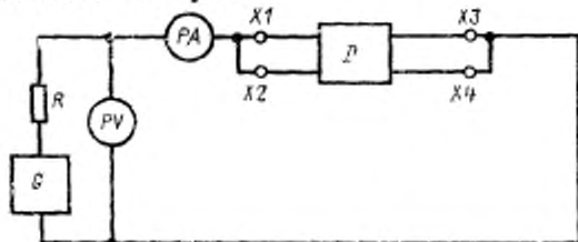
G—источник постоянного напряжения; R—защитное сопротивление; PV—измеритель постоянного напряжения; PA—измеритель постоянного тока; X1, X2, X3, X4—выводы прибора; D—проверяемый прибор.
