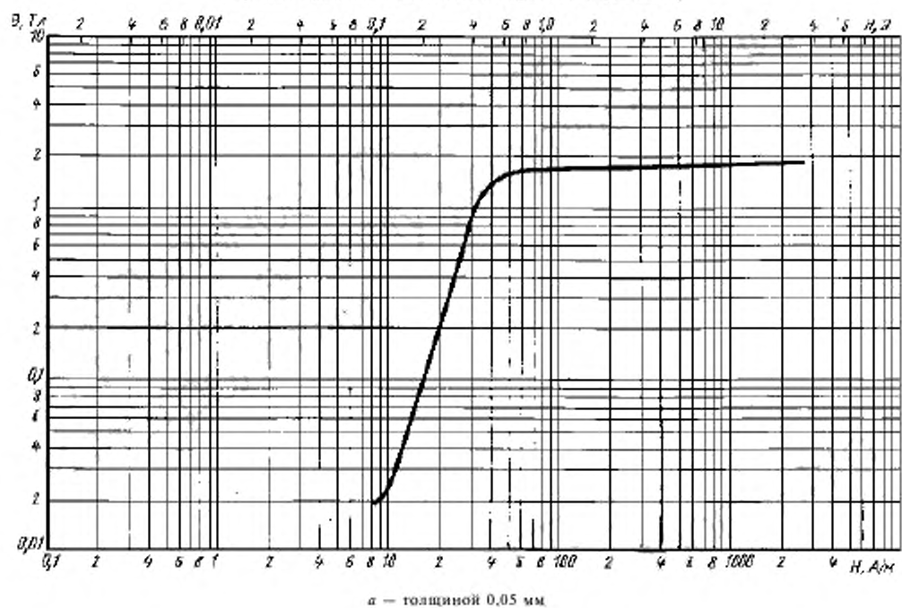
Кривые намагничивания стали марки 3425 (Э360АА)
