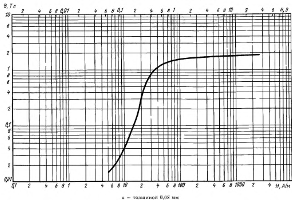
Кривые намагничивания стали марки 3424 (Э360А)
