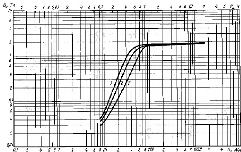
Кривые намагничивания стали марки 3425 (Э360АА) для частот: 1 — 400 Гц, 2 — 1000 Гц, 3 — 3000 Гц
