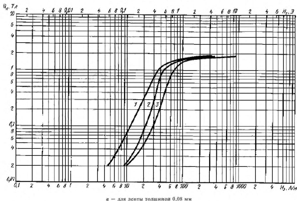
Кривые намагничивания стали марки 3424 (Э360А) для частот: 1 — 400 Гц, 2 — 1000 Гц, 3 — 3000 Гц
