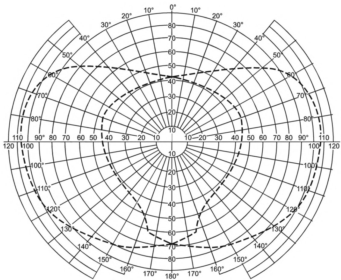
Рисунок 2 — Диаграмма апертометра
