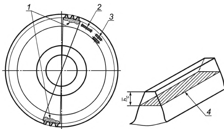
1 — поперечный темплет; 2 — один образец на растяжение по ГОСТ 1497, тип III; 3 — два образца на ударную вязкость при температуре 20 °С по ГОСТ 9454, тип 1; 4 — продольный темплет
