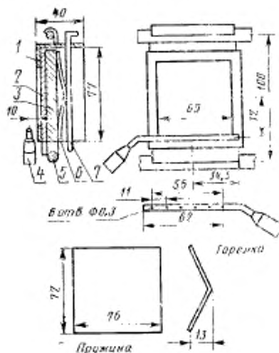
1 — корпус держателя образца; 2 — образец; 3 — прижимная пластина из асбестовой плиты толщиной 10 мм; 4 — горелка; 5 — опорные стержни; 6 — пружина из фосфористой бронзы толщиной 0,8 мм; 7 — штырь из стальной проволоки диаметром 3 мм
