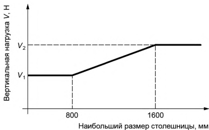
Рисунок 8 — Определение устойчивости под действием вертикальной нагрузки
