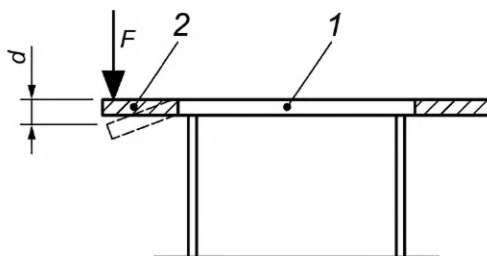
Рисунок 5 — Испытание под действием вертикальной статической нагрузки — дополнительная поверхность
