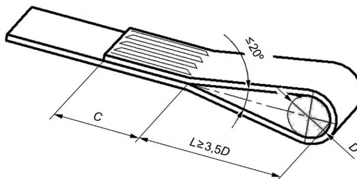
Рисунок 15 — Допустимый угол в петле стропа при соединении с концевым элементом
