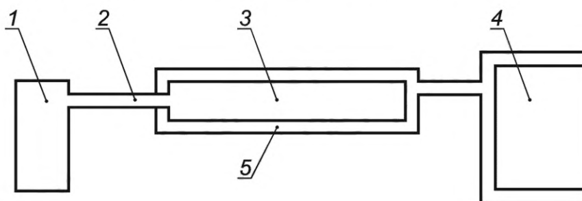
1 — газ; 2 — внешнее подключение для контроля P_g ; 3 — трубки в сборе; 4 — масс-спектрометр для обнаружения утечек методом глобального вакуума; 5 — климатическая камера
