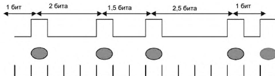
Рисунок 2 – Структура синхронизирующей метки
