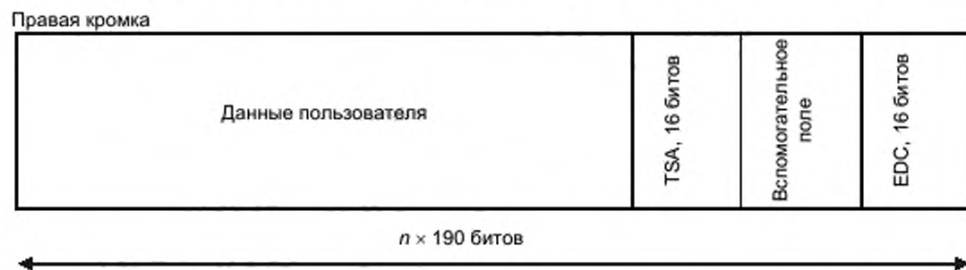
Рисунок 10 – Структура блока данных сектора (за исключением секторов типа 5)
