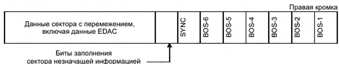
Рисунок 8 – Структура сектора, типы 0 – 5
