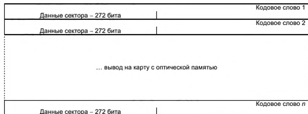
Рисунок 14 – Перемежение данных сектора, сектор типа 5
