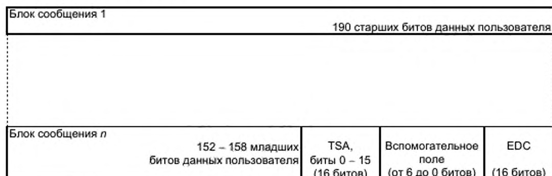
Рисунок 12 – Данные сектора до применения кода EDAC (для секторов всех типов, за исключением типа 5)
