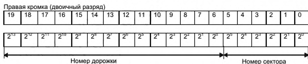
Рисунок 4 – Формат адреса сектора и дорожки
