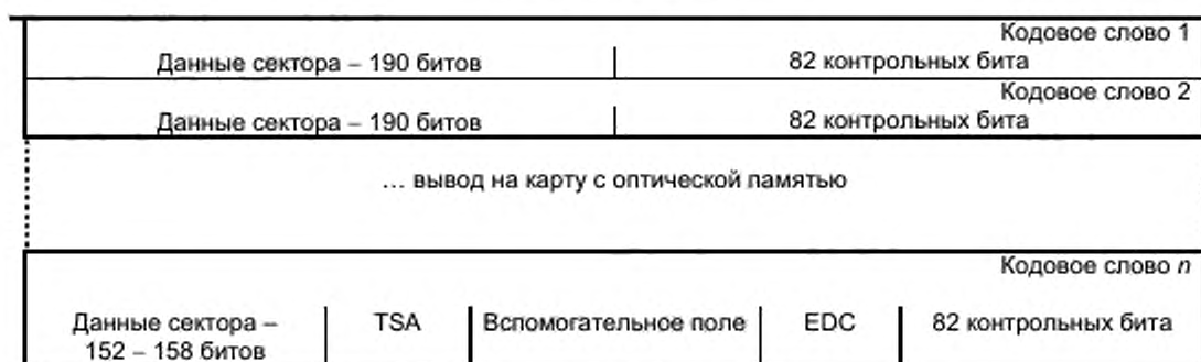
Рисунок 13 – Перемежение данных сектора с кодом EDAC, секторы типов 0 – 4
