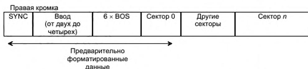
Рисунок 6 – Структура дорожки с неполной записью, секторы типов 0 – 5
