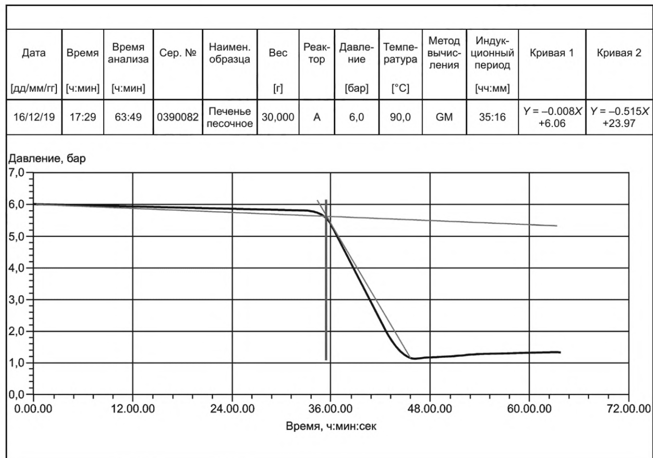
Рисунок В.2 — Барометрическая кривая индукционного периода печеня, полученная оператором методом наименьших квадратов
