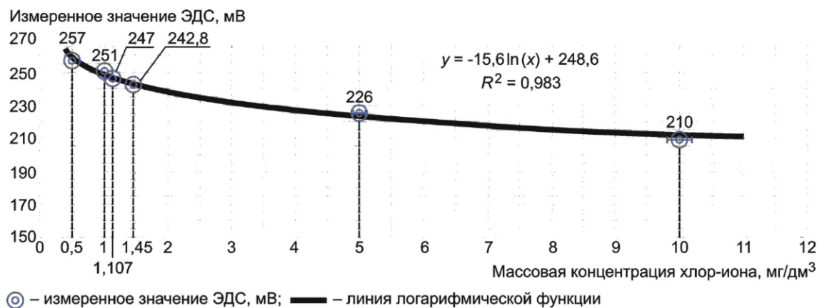
Рисунок В.1 — Зависимость ЭДС (мВ) от концентрации хлор-иона (мг/дм³)
