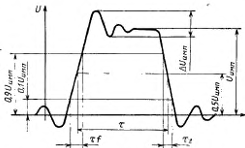
\tau — длительность импульса; \tau_f — длительность фронта импульса; \tau_s — длительность спада импульса; U_{имп} — амплитуда импульса; \Delta U_{имп} — неравномерность вершины импульса, включая выбросы на вершине импульса
