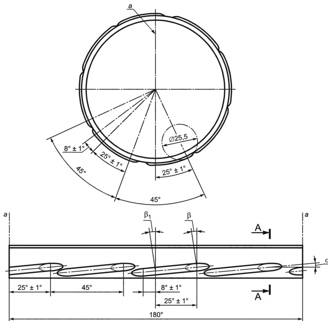
Рисунок 2 — Конструкция и увеличенные детали резьбы
