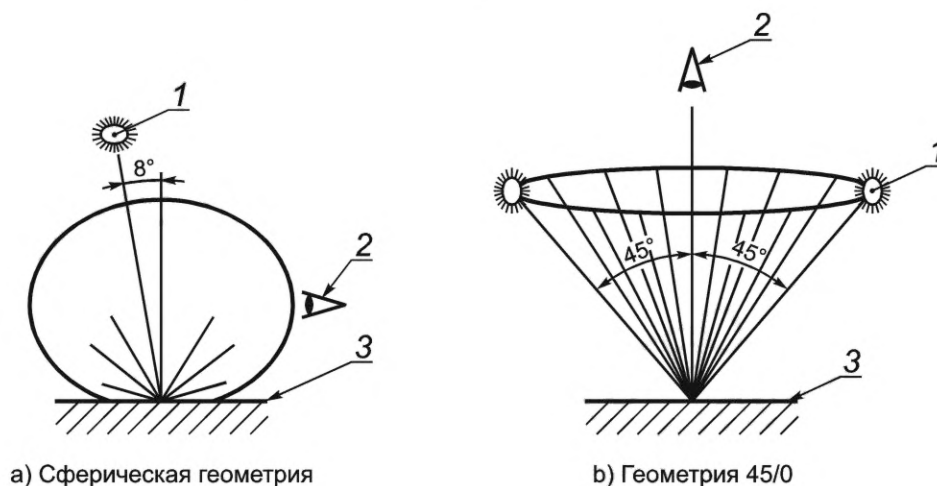
Рисунок 1 — Пример отраженного излучения для спектрофотометров с геометрией измерения 8/d и 45/0
