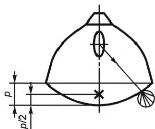
г – рассеиватель выпуклый матированный или призматический
