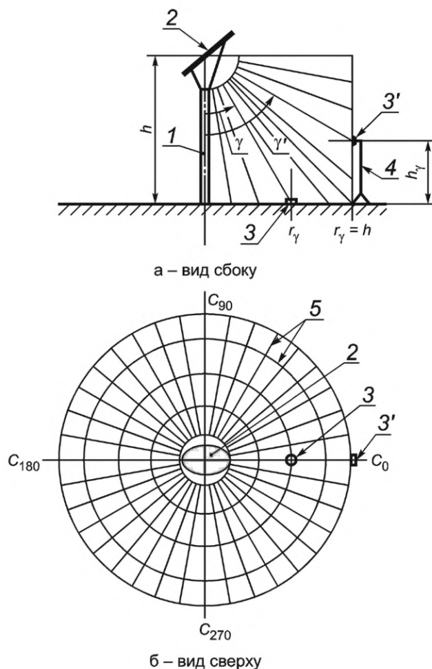
1 — стойка осветительного устройства; 2 — отражающий экран; 3 и 3' — фотометрическая головка в положении измерения горизонтальной и вертикальной освещенности соответственно; 4 — раздвижной штатив; 5 — измерительная сетка горизонтальной плоскости в системе фотометрирования C, \gamma
