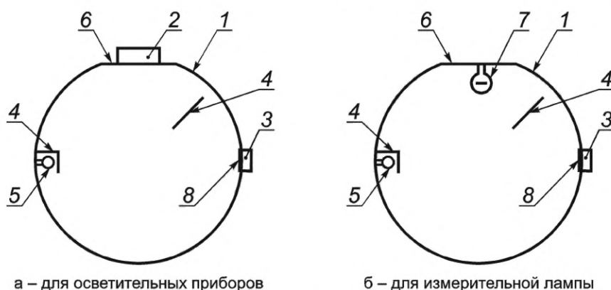
Рисунок 3 — Схема измерения в фотометрическом шаре светового потока осветительного прибора с плоским выходным отверстием
