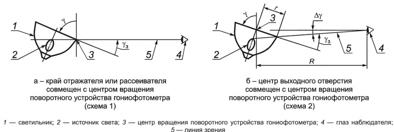
Рисунок 5 — Визуальный способ определения защитного угла светильника
