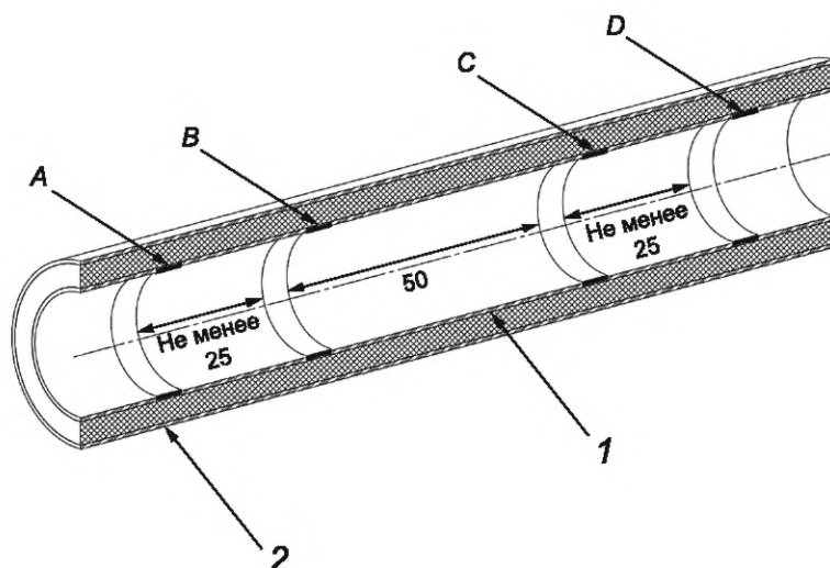
A и D — токовые электроды; B и C — потенциальные электроды; 1 — экран по жиле; 2 — экран по изоляции
