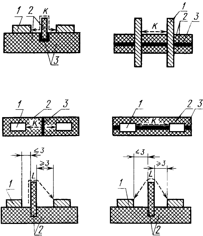
L — электрический зазор; K — путь утечки; 1 — металл; 2 — электроизоляционный материал; 3 — клеевое соединение
