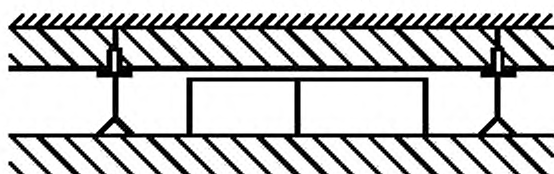
с - Система кабельных или специальных кабельных коробов, предназначенная для установки под полом (установлена внутри двоякого пола)
