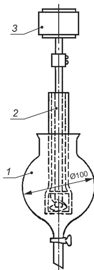
1 — круглая делительная воронка; 2 — мешалка; 3 — электродвигатель
