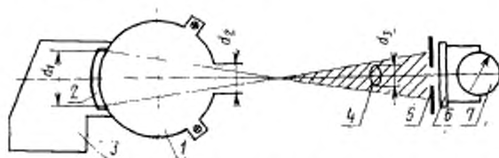
1—фотометрический шар; 2—сменные кольцевые сегменты; 3—внутренний черный предмет; 4—объектив; 5—диафрагма фотоприемника; 6—фотоприемник; 7—измерительный прибор
