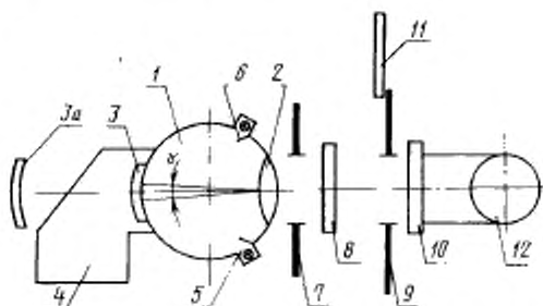
1—фотометрический шар; 2—коллиматорный объектив; 3—кольцевой сегмент; 3а—сплошной сегмент; 4—имитатор черного предмета; 5—источник света; 6—заслонки; 7—диафрагма шара; 8—испытываемое изделие; 9—диафрагма фотоприемника; 10—фотоприемник; 11—матовое стекло; 12—измерительный прибор
