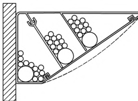
б) СКК/ССКК поперечного сечения, отличного от прямоугольного
