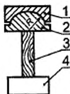
1, 2 — самоустанавливающиеся пластины; 3 — образец; 4 — нижняя платформа испытательной машины
