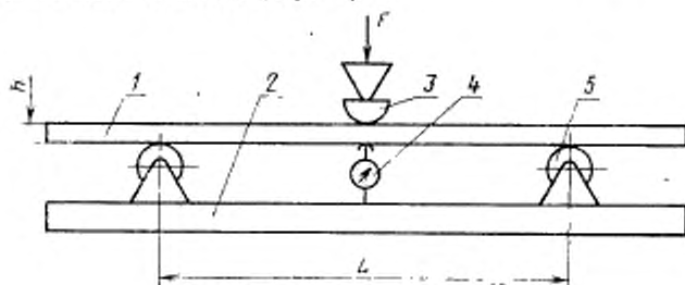
1 - образец; 2 - основание; 3 - нагружающий элемент; 4 - прибор для измерения прогиба; 5 - опоры
