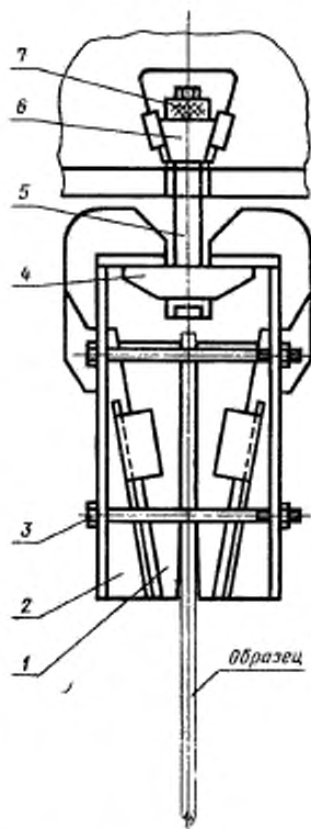
1—губка; 2—скоба; 3—болт; 4—основание; 5—тяги; 6—сухари; 7—гайка
