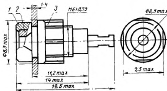
Гнездо Г1,6
