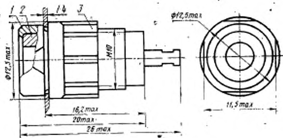
Гнездо Г4,0
