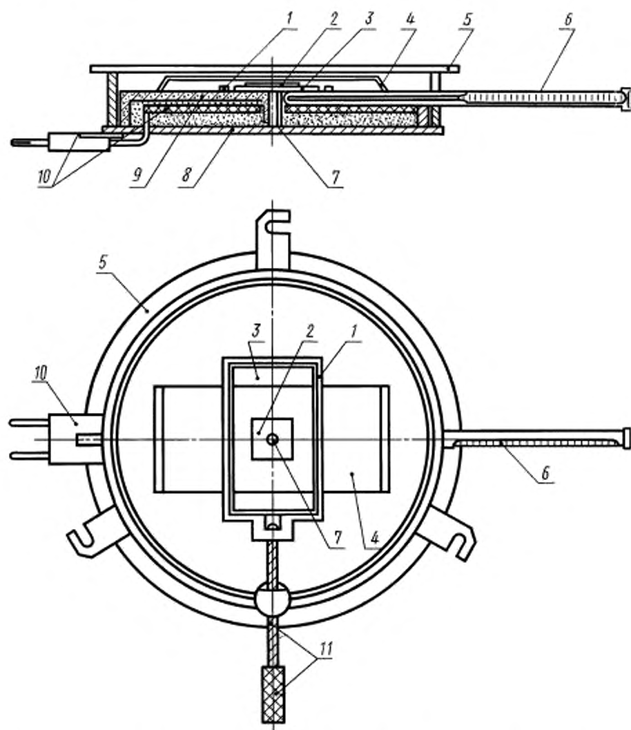
1 — подвижная рамка; 2 — покровное стекло; 3 — предметное стекло; 4 — тепловой экран; 5 — крышка; 6 — термометр; 7 — отверстие для прохода света; 8 — камера; 9 — металлический блок; 10 — электронагре- ватель с регулятором; 11 — микрометрический винт
