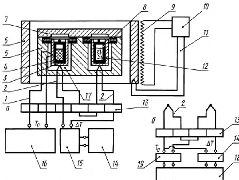
1 — термпара для измерения температуры ячейки с образцом ( T_0 ); 2 — дифференциальная термпара ( \Delta T ); 3 — ячейка-держатель образца; 4 — съемный стаканчик для образца; 5 — нагреваемый блок; 6 — термокамера; 7 — крышка блока; 8 — съемный стаканчик для эталона; 9 — нагреватель; 10 — регулятор; 11 — датчик регулятора; 12 — ячейка-держатель эталона; 13 — блок «холодных» спаев термпар; 14 — регистратор \Delta T ; 15 — фотокомпенсационный усилитель сигнала \Delta T ; 16 — регистратор T_0 ; 17 — гнезда; 18 — регистратор T_0 , \Delta T ; 19 — компенсатор сигнала T_0
