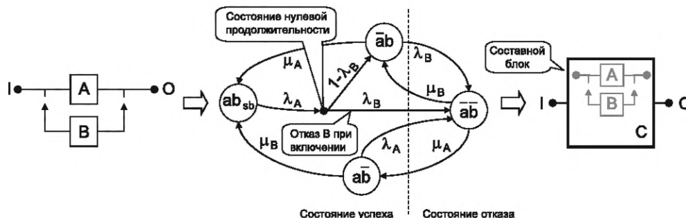
Рисунок 23 — Резервирование замещением
