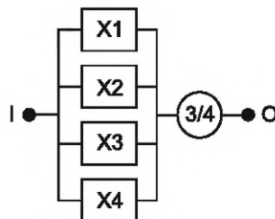
Рисунок 9 — Структура резервирования 3 из 4
