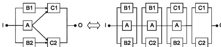
Рисунок 19 — Эквивалентные RBD с минимальными наборами обрывов
