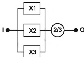
Рисунок 8 — Структура резервирования 2 из 3
