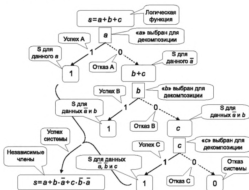
Рисунок 33 — Декомпозиция Шеннона, эквивалентная таблице 5
