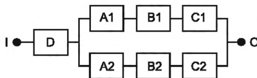
Рисунок 6 — Общая последовательно-параллельная структурная схема надежности
