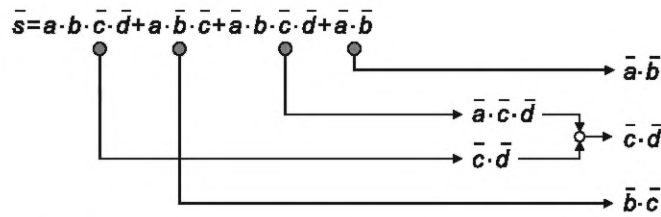
Рисунок В.12 — Определение путей отказа (наборов обрывов) по RBD
