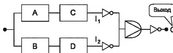
Рисунок 49 — Применение вентиль PAND
