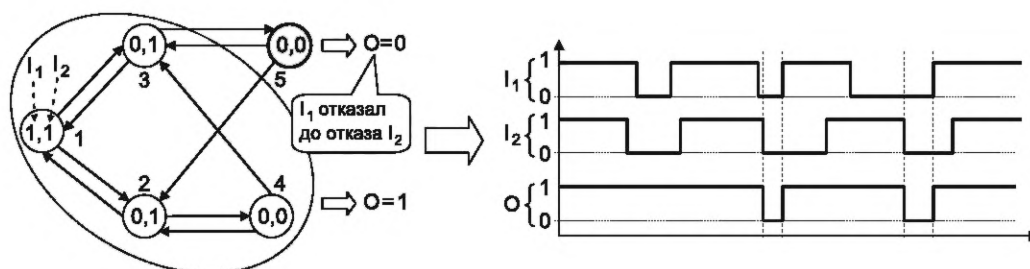
Рисунок 50 — Эквивалентный конечный автомат и пример его хронограммы для вентиль PAND
