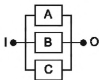
Рисунок 32 — RBD системы из трех резервированных объектов
