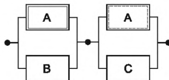
Рисунок 43 — Пример RBD с блоками в прямом и обратном состояниях
