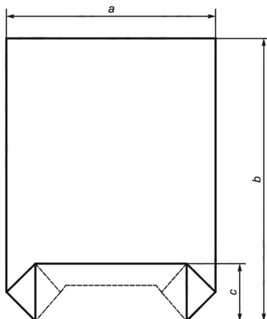
Рисунок 1 — Мешок типа I — коробчатый с открытым верхом
