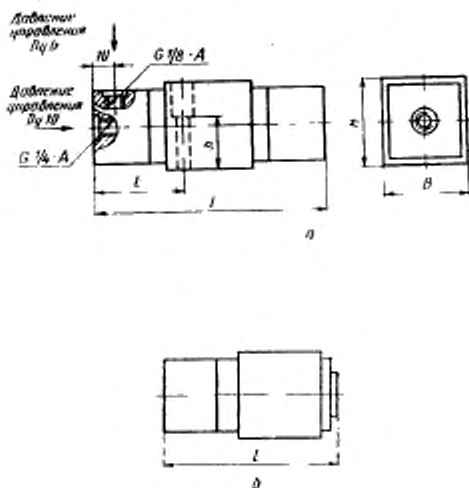
а — с двумя пневмоголовками; б — с одной пневмоголовкой
