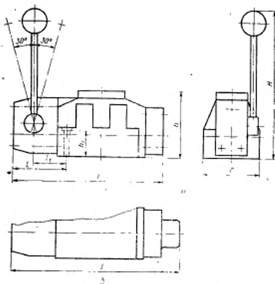
а — трехпозиционный; б — двухпозиционный
