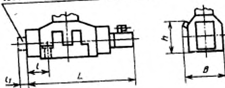
Узел настройки хода золотника
