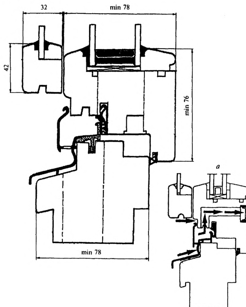
Рисунок 2 — Примеры конструктивного решения оконного блока спаренной конструкции на базе конструкции по ГОСТ 24700 (нижний притвор)
