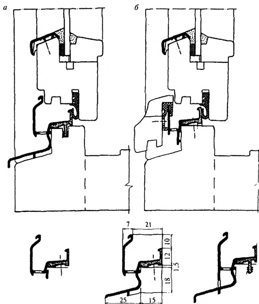
Рисунок 12 — Примеры конструкций дождезащитных профилей: а — из алюминиевых сплавов с термовставкой; б — то же, с деревянной наружной облицовкой
