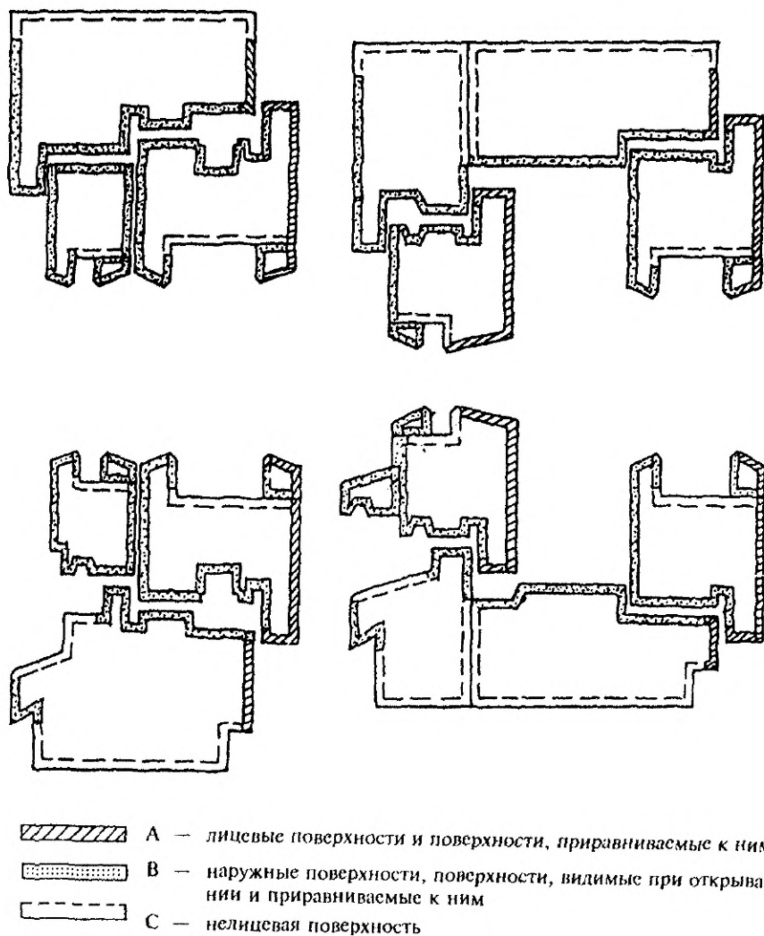
Рисунок 8 — Примеры определения видов поверхностей деталей
