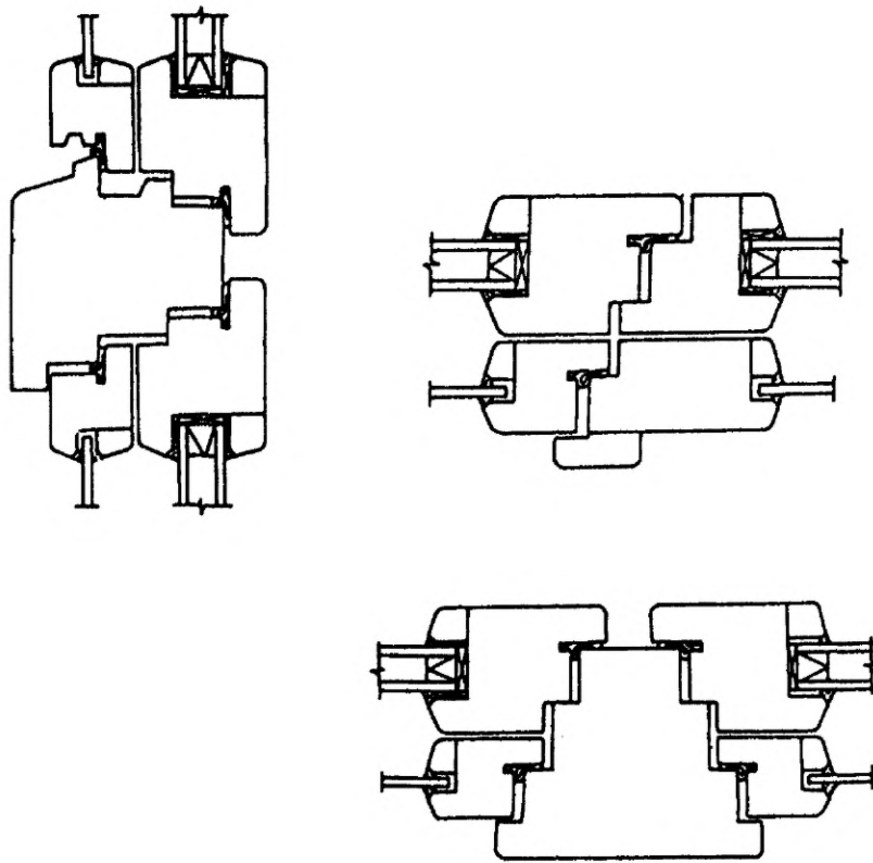
Рисунок 3 — Примеры конструктивных решений импостных и безимпостных притворов оконных блоков спаренной конструкции (вариант распашного открывания)
