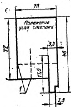
1 — точки подвеса грузов
