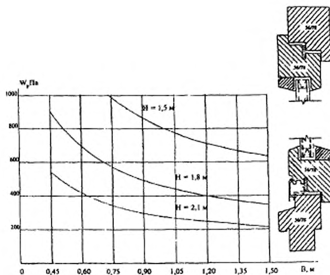
Рисунок Б.1 — Пример графического определения соотношения высоты H и ширины B створчатых элементов с сечением брусков 56 х 78 мм в случае воздействия ветровой нагрузки W_p (для распашного и поворотного-откидного открывания, масса стеклопакета — не более 50 кг)
