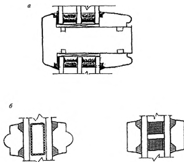
a — брусок горбылькового переплета; б — накладные декоративные раскладки (ложные горбыльки)
