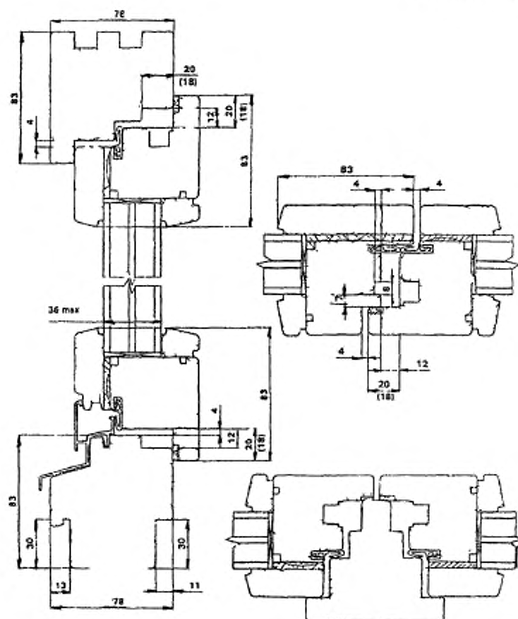
Рисунок 1 — Пример конструктивного решения оконного блока
