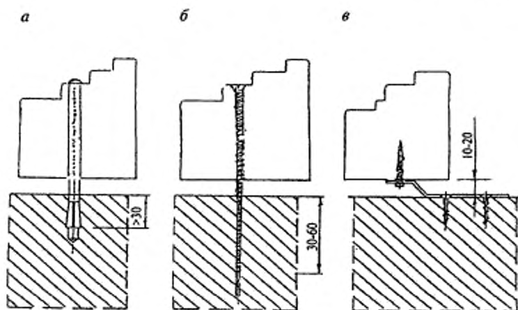
a — узел крепления стропильным дюбелем; б — узел крепления монтажным шурупом; в — узел крепления при помощи анкерной пластины
