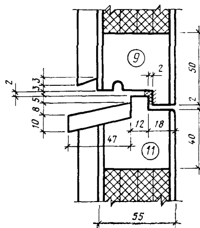
г) По среднему притвору
