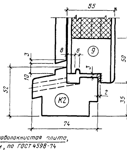
б) По нижнему притвору
