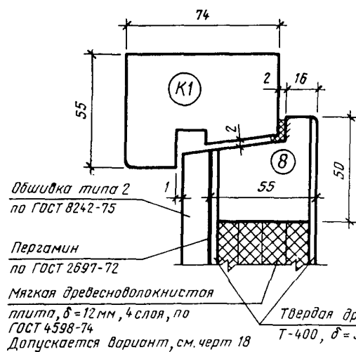
а) По верхнему притвору
