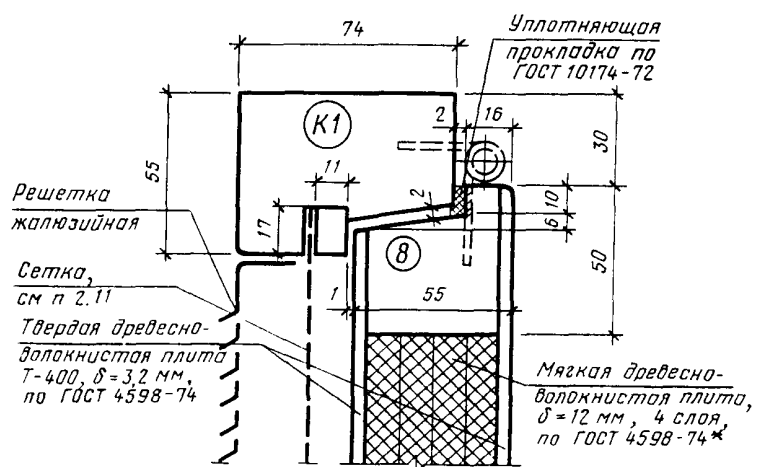
Сечение А6
