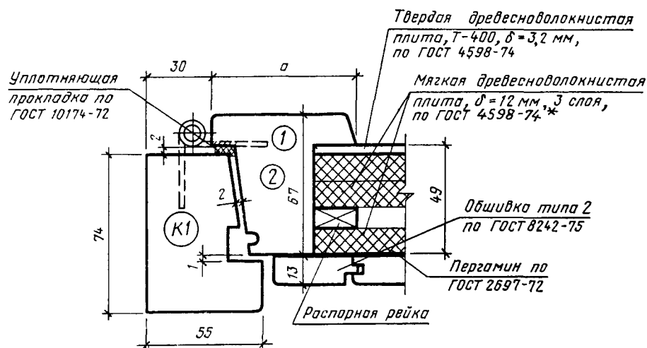
Сечения А10 и Б5
