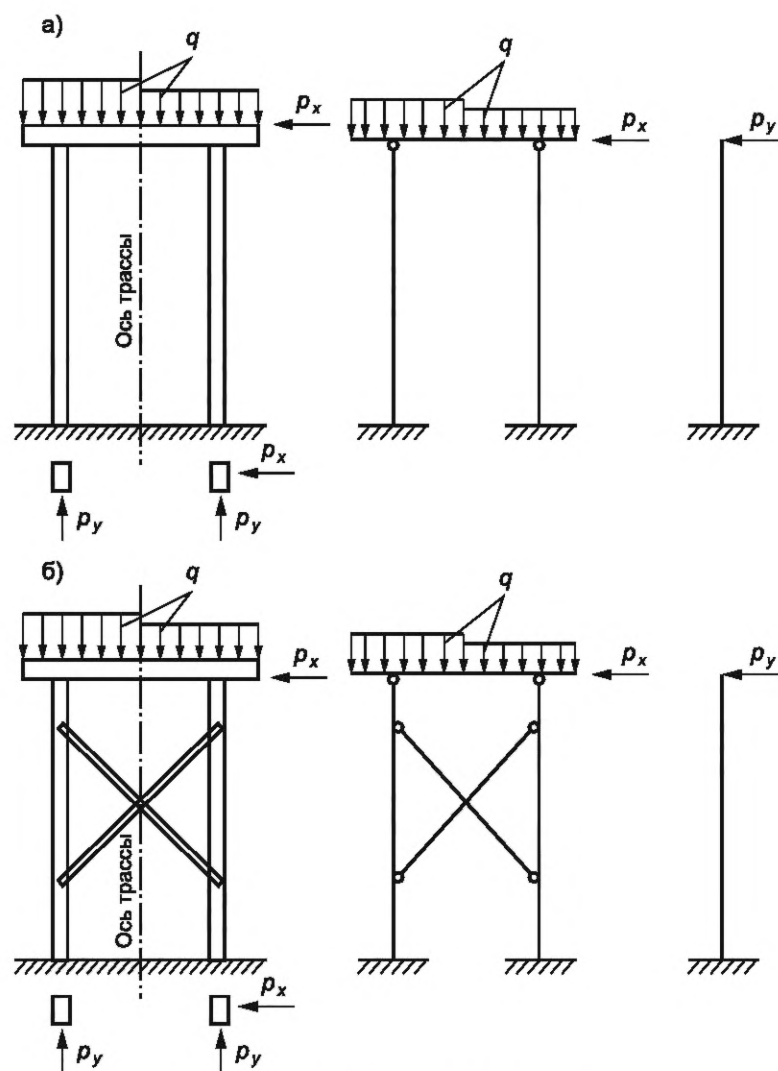
Рисунок А.14 — Расчетные схемы железобетонных опор
