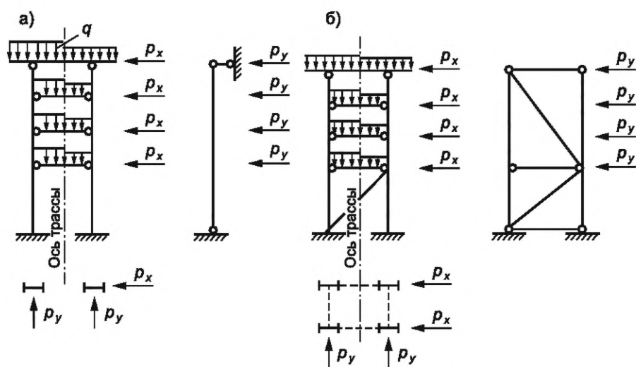
Рисунок А.15 — Расчетные схемы стальных многоярусных опор
