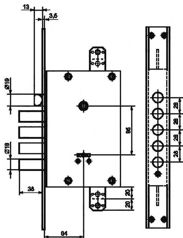
Рисунок Б.6 — Пример сувальдного врезного замка типа 3Б11
