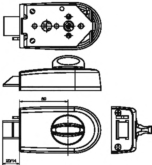
Рисунок Б.9 — Пример накладного замка типа 3НЗ с засовом-защелкой
