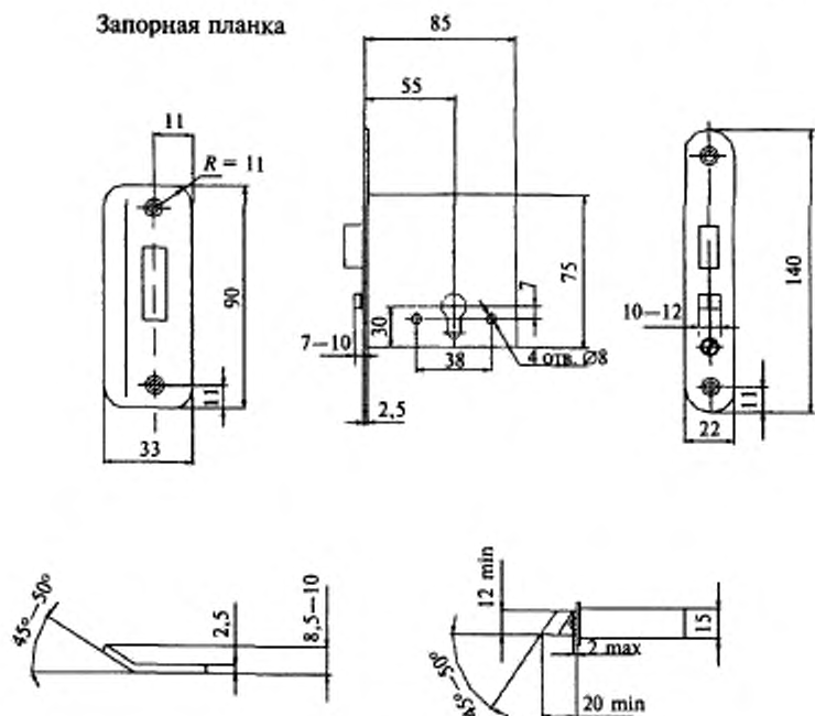
Рисунок В.5 — Пример замка врезного цилиндрического типа ЗВ2 с автоматическим выводом засова-защелки
