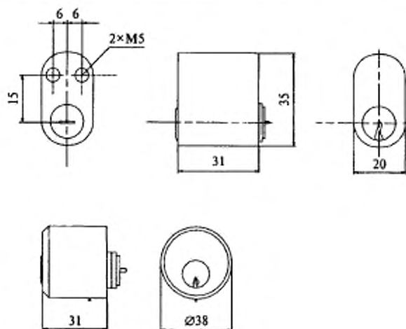
Рисунок В.25 — Примеры механизмов цилиндрических односторонних для врезных замков, тип МЦЗ
