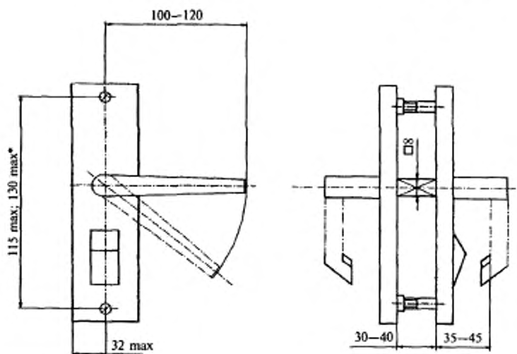
Рисунок В.36 — Пример ручек фалевых с накладками для защелок, тип РФ5
