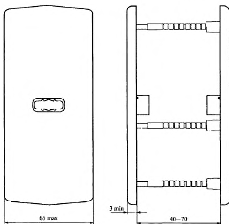
Рисунок В.41 — Пример защитной накладки
