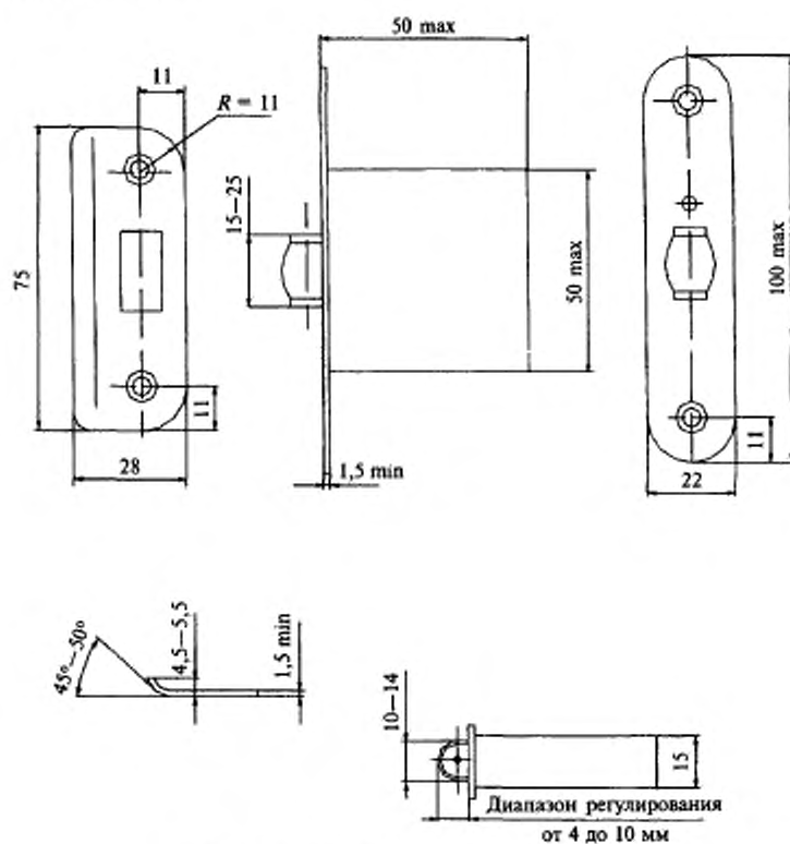
Рисунок В.22 — Пример зашелки врезной типа ЗЩ4
