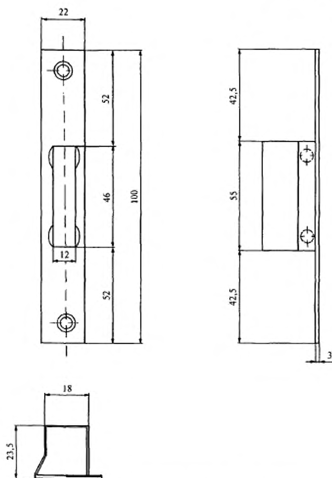
Рисунок В.43 — Пример коробчатой запорной планки
