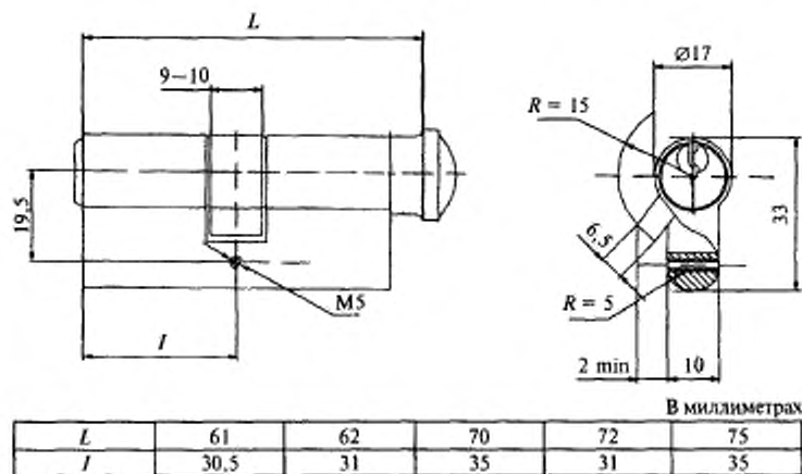
Рисунок В.24 — Пример механизма цилиндрического пластинчатого одностороннего с постоянным ключом для врезных замков, тип МЦ2
