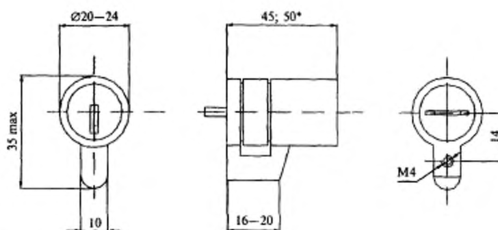
Рисунок В.29 — Пример механизма цилиндрического пластинчатого для накладных замков, тип МЦ9
