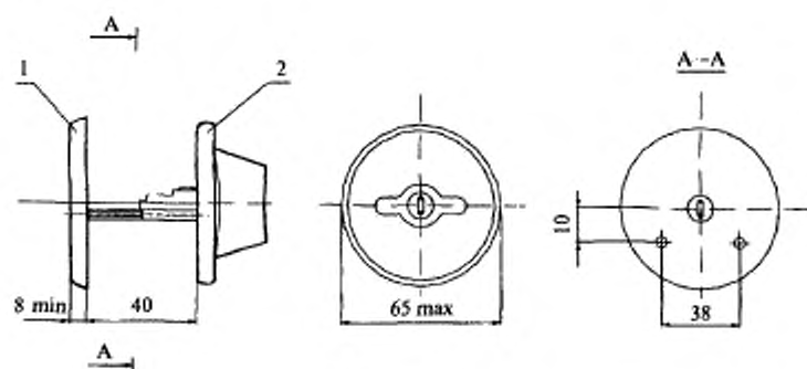
Рисунок В.39 — Пример накладок для врезных замков с цилиндрическим механизмом МЦ4, тип Н2
