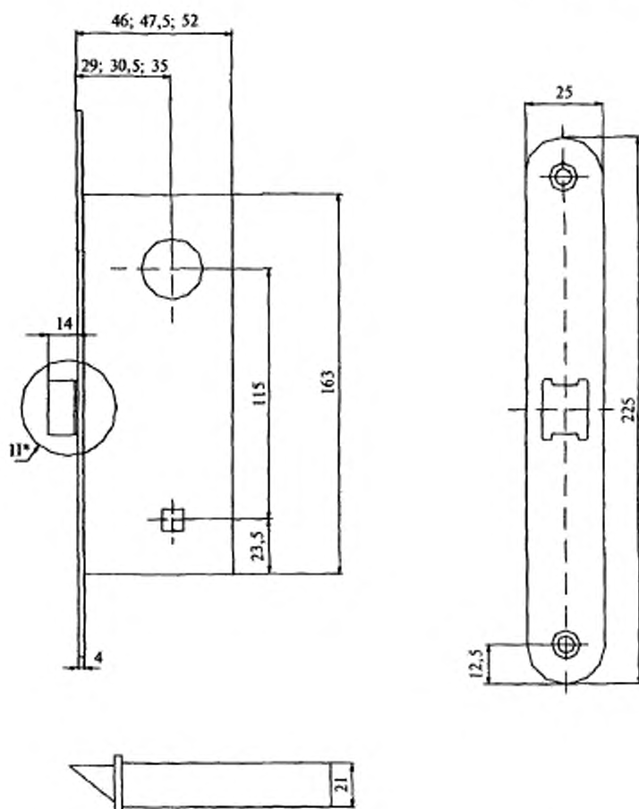
Рисунок В.11 — Пример замка врезного цилиндрического типа ЗВ4 для дверных блоков из поливинилхлоридных или алюминиевых профильных деталей
