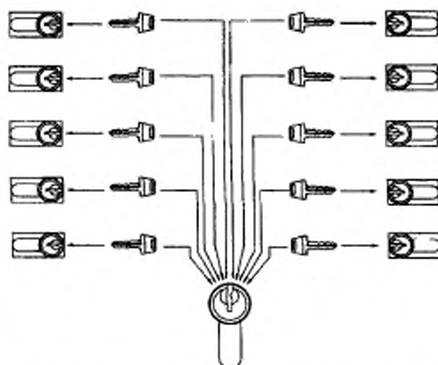
Рисунок Б.5 — Система цилиндрических механизмов с центральным механизмом — группа цилиндрических механизмов, включающая механизм, который можно открывать и закрывать ключами, свойственными для каждого из механизмов этой группы
