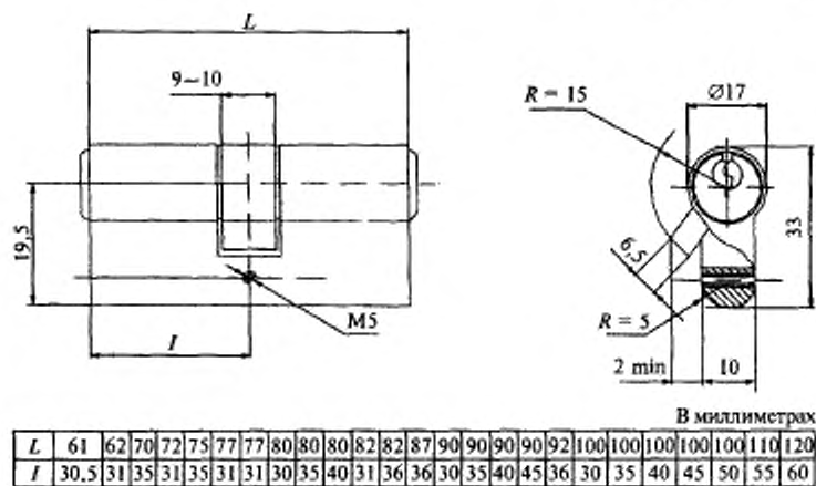
Рисунок В.23 — Пример механизма цилиндрического штифтового двухстороннего для врезных замков, тип МЦ1
