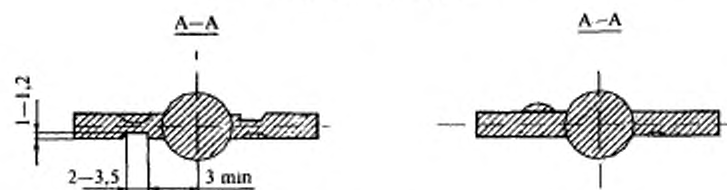
Рисунок В.46 — Пример ключа для врезного сувальдного замка, тип 3C1
