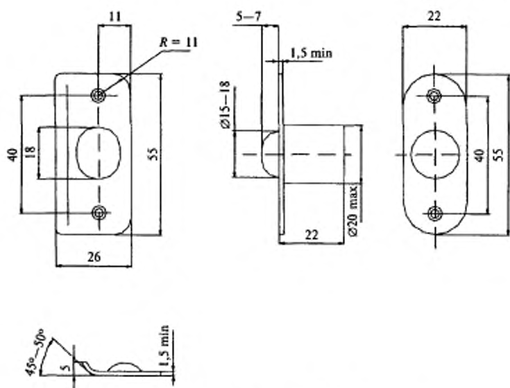
Рисунок В.21 — Пример зашелки врезной типа ЗЩЗ
