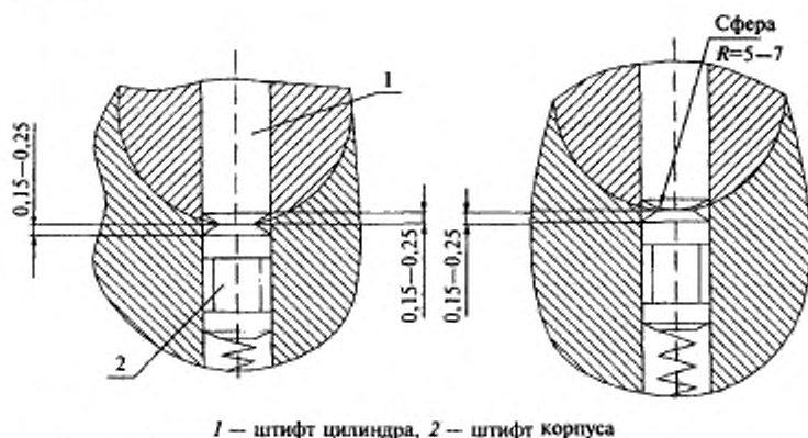
1 — штифт цилиндра, 2 — штифт корпуса Рисунок 1 — Примеры фасок и сфер штифтов цилиндра и корпуса цилиндрического механизма
