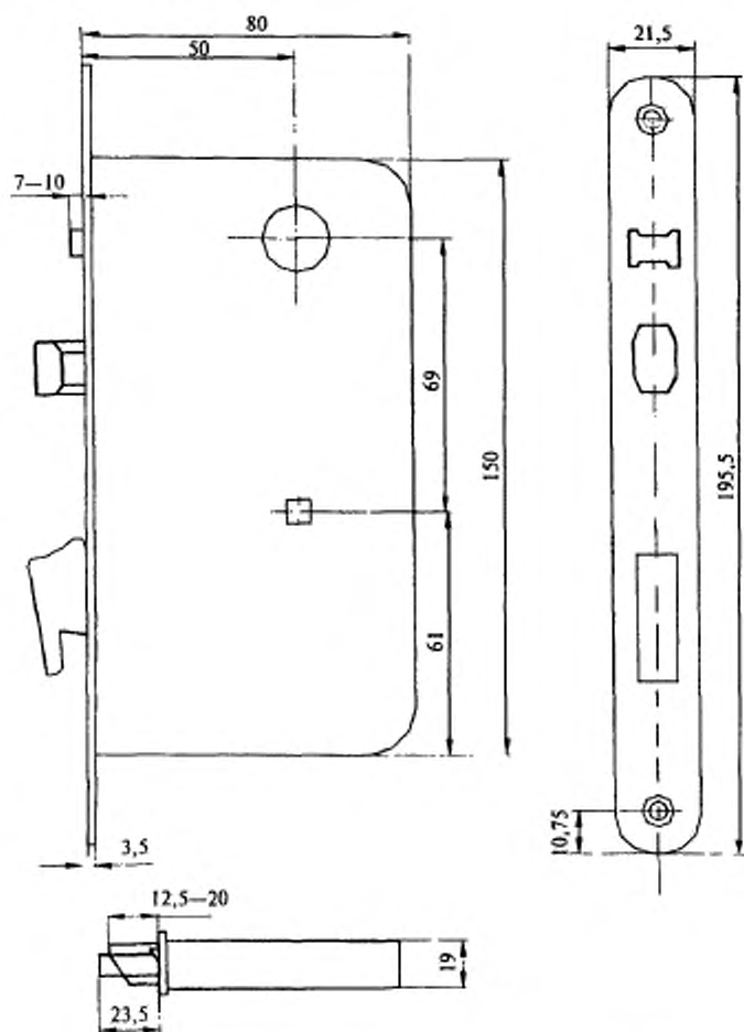
Рисунок В.8 — Пример замка врезного цилиндрического типа ЗВ7 с крюкообразным засовом и автоматическим выводом засова-заселки
