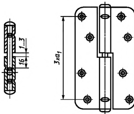
Типоразмеры ПНЗ-110, ПНЗ-130, ПНЗ-150
