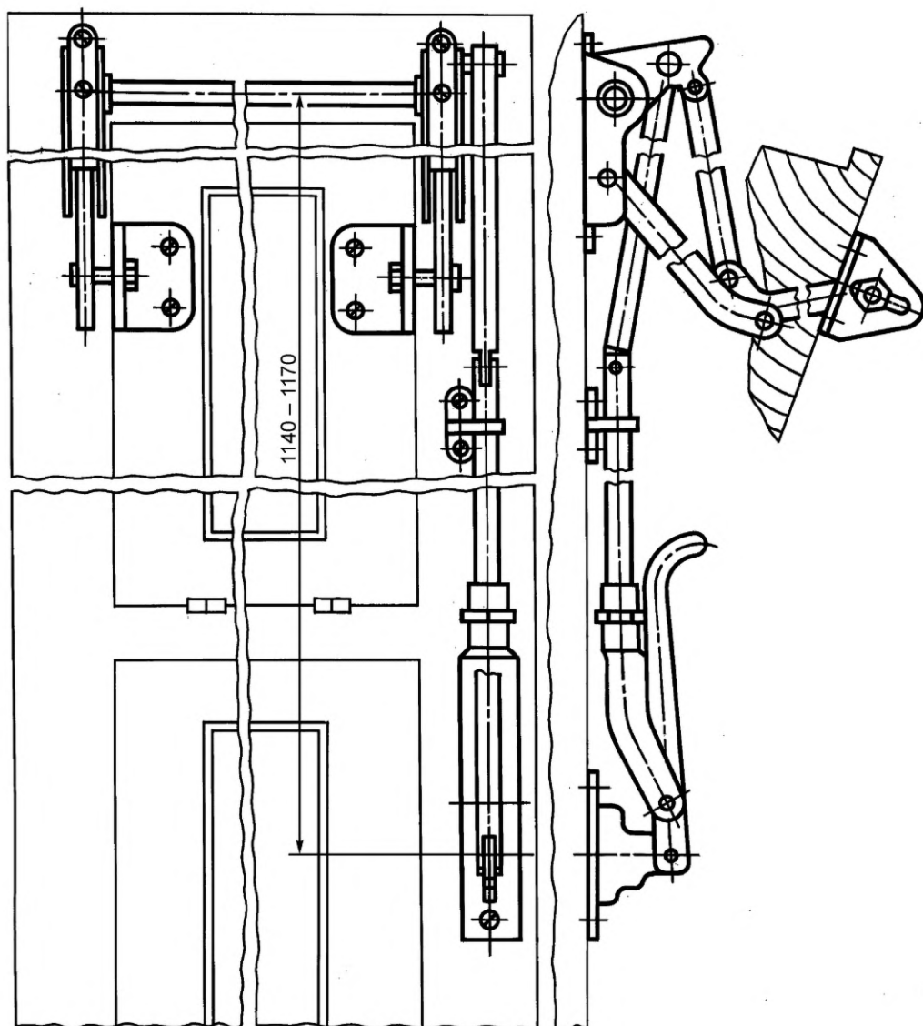
Рисунок В.1 — Фрамужный прибор типа ПФ-1
