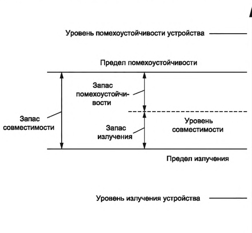
Рисунок 3 — Принцип ЭМС
