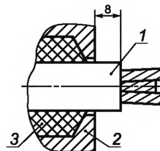
1 — оболочка кабеля; 2 — стенка вводного устройства; 3 — уплотнение
