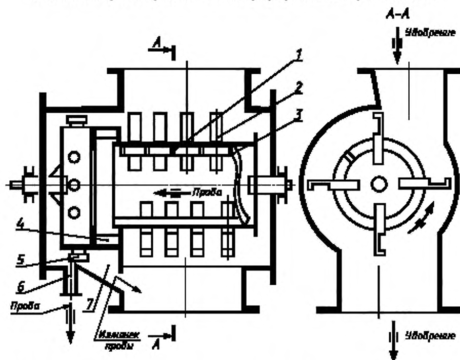
1 — полый цилиндрический ротор; 2 — заборный поворотный желобок; 3 — спиральные направляющие полосы; 4 — смесительная камера; 5 — делитель пробы; 6 — точка отбора пробы; 7 — точка излишка пробы
