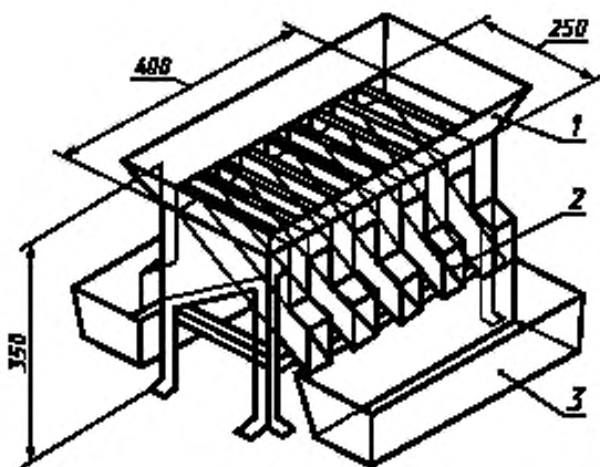
1 — бункер; 2 — течка; 3 — приемник
