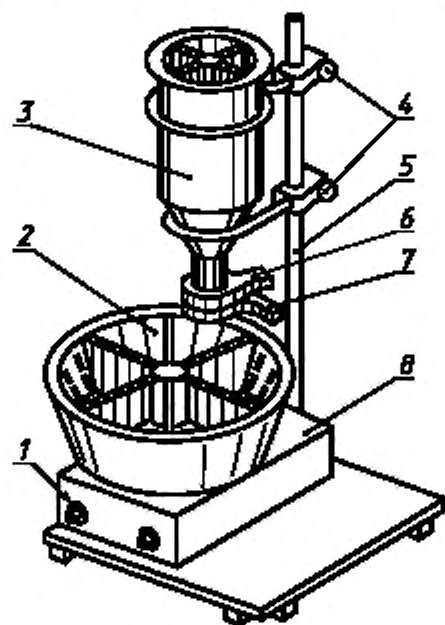
1 — включатель; 2 — делитель; 3 — усреднитель; 4 — держатель; 5 — штанга; 6 — отсекающий; 7 — диа- фрагма; 8 — электродвигатель
